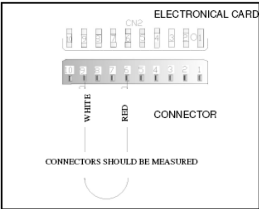
Contacts CN2.6 et CN2.9
